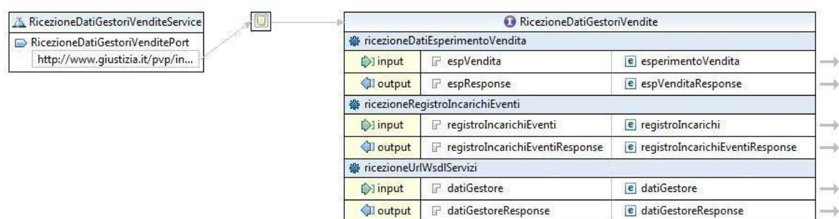
Figura 20 WSDL ricezione dati Gestore delle Vendite
