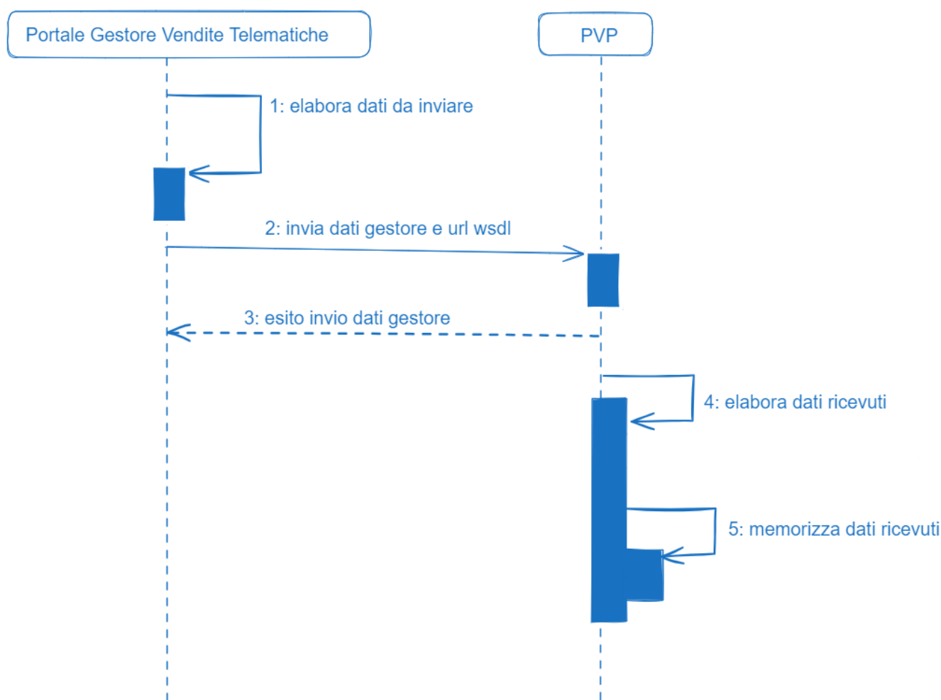
Figura 10 Modalità operativa trasmissione URL WSDL dei servizi esposti dal Gestore delle Vendite
