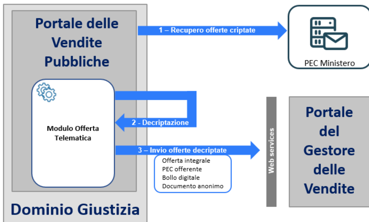
Figura 3 Decriptazione ed invio offerte
