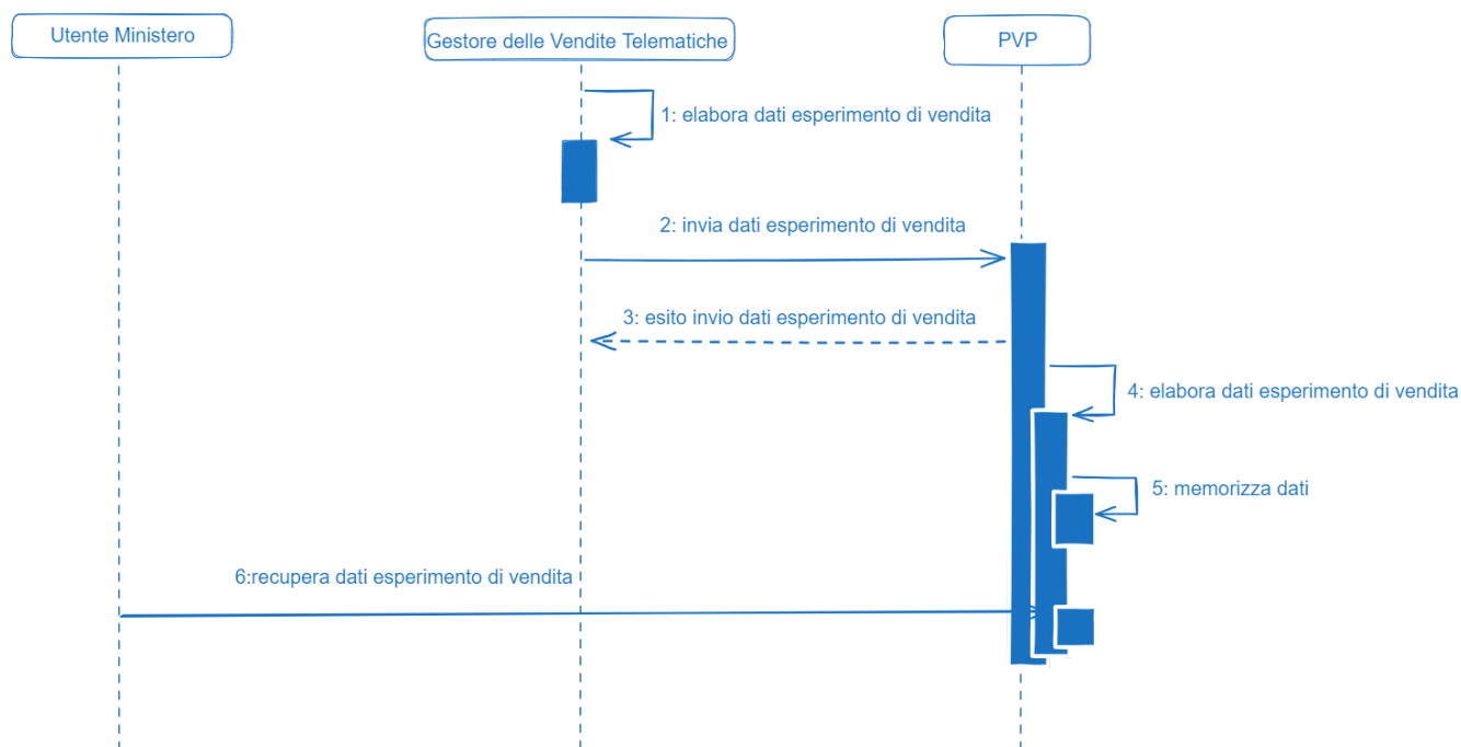
Figura 7 Modalità operativa trasmissione dati esperimento vendita
