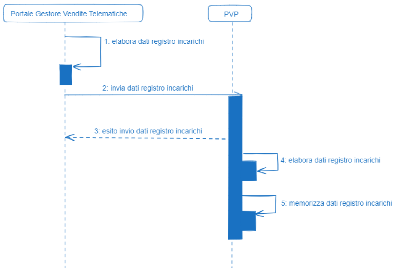
Figura 8 Modalità operativa trasmissione dati registro incarichi
