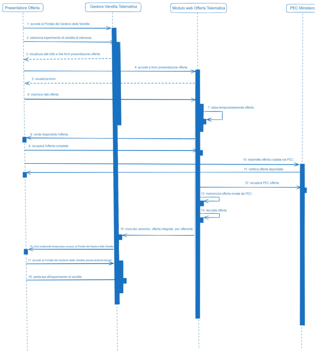
Figura 6 Modalità operativa trasmissione offerta telematica
