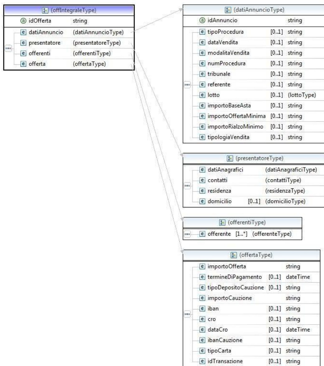
Figura 12 Relazioni tra offerIntegraleType e le strutture principali
