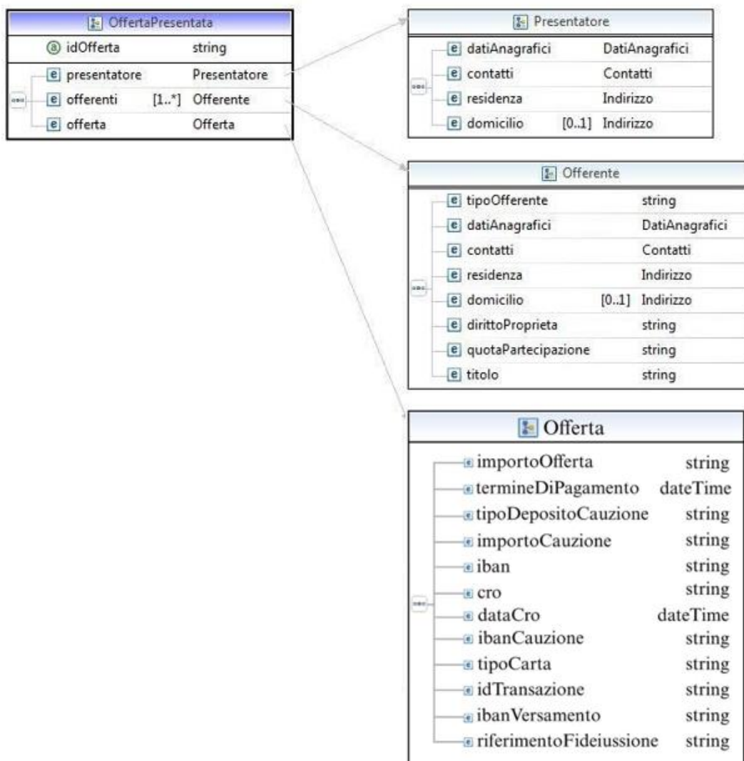
Figura 24 Relazioni tra OffertaPresentata e le strutture Presentatore, Offerente e Offerta
