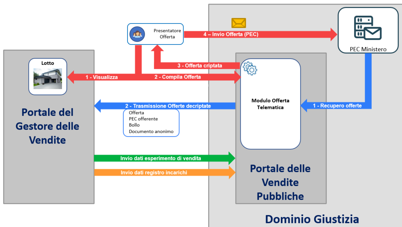
Figura 1 Architettura generale
