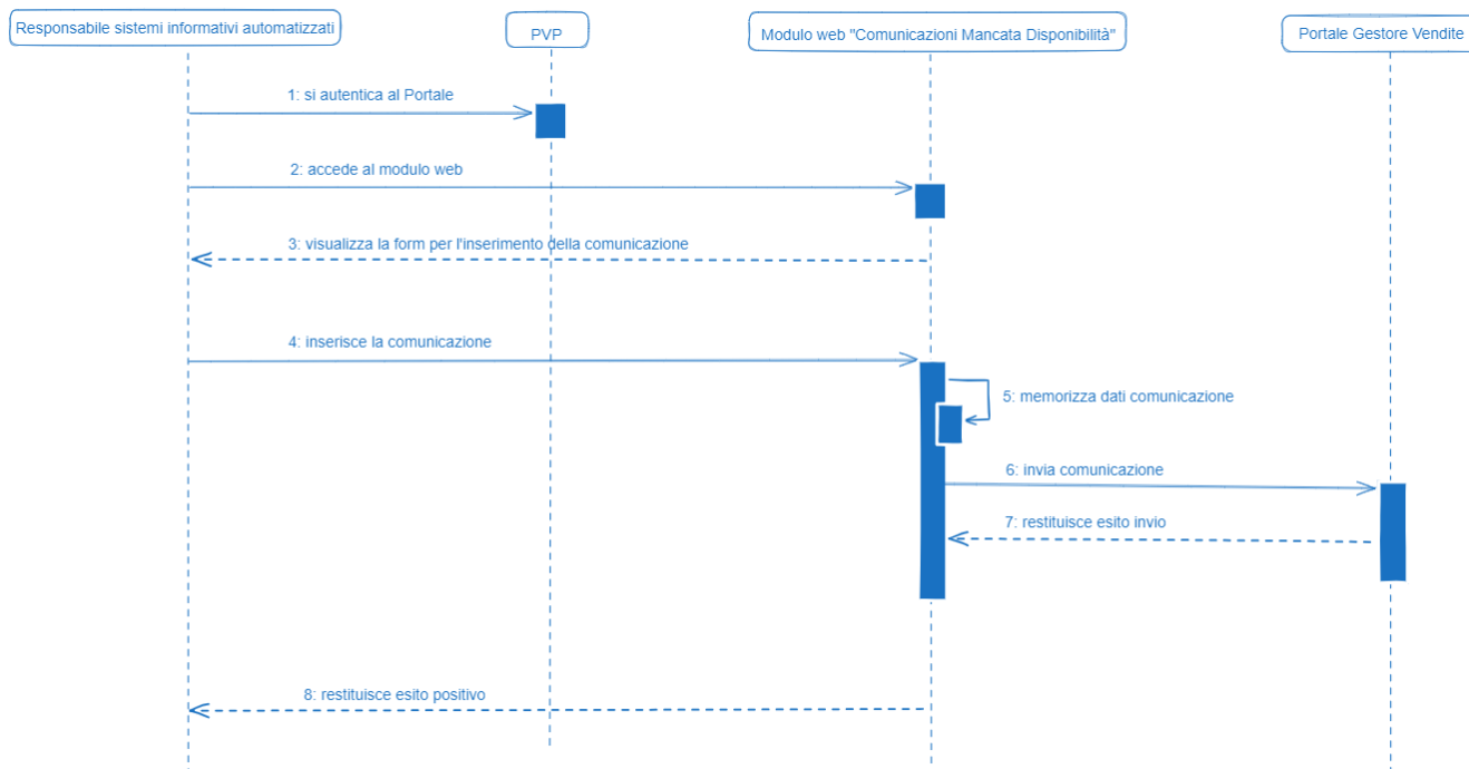
Figura 9 Modalità operativa trasmissione mancata disponibilità programmata
