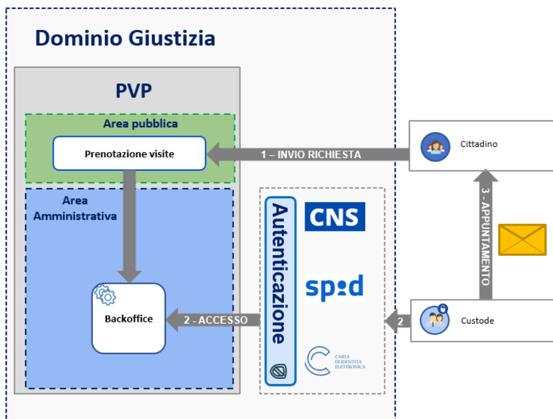
Figura 4 – Richiesta visita immobile
