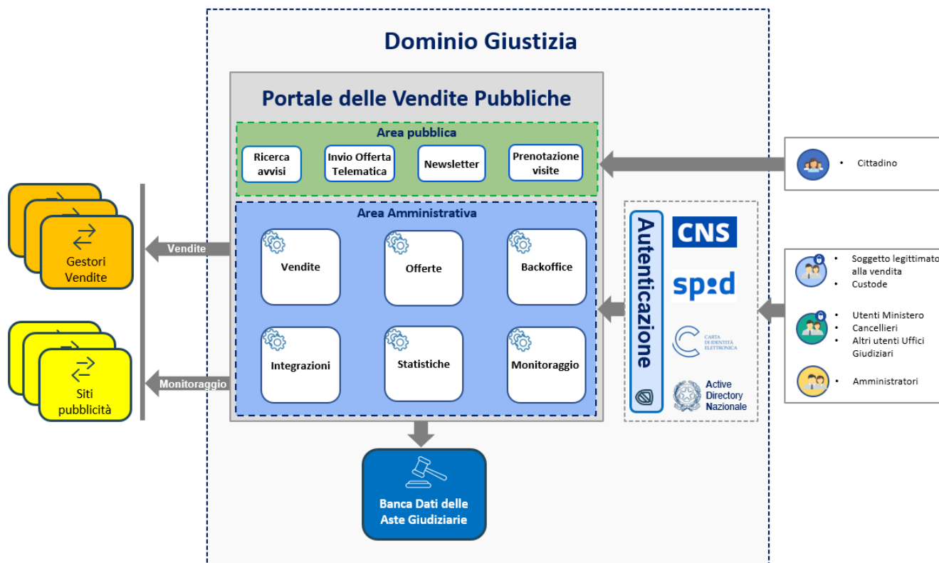
Figura 1 - Architettura generale del sistema
