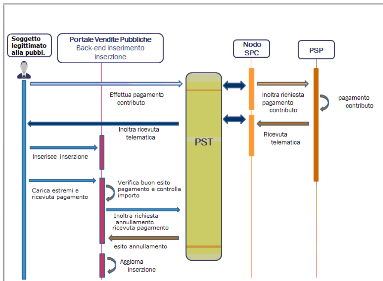
Figura 7 pagamento contributo pubblicazione
