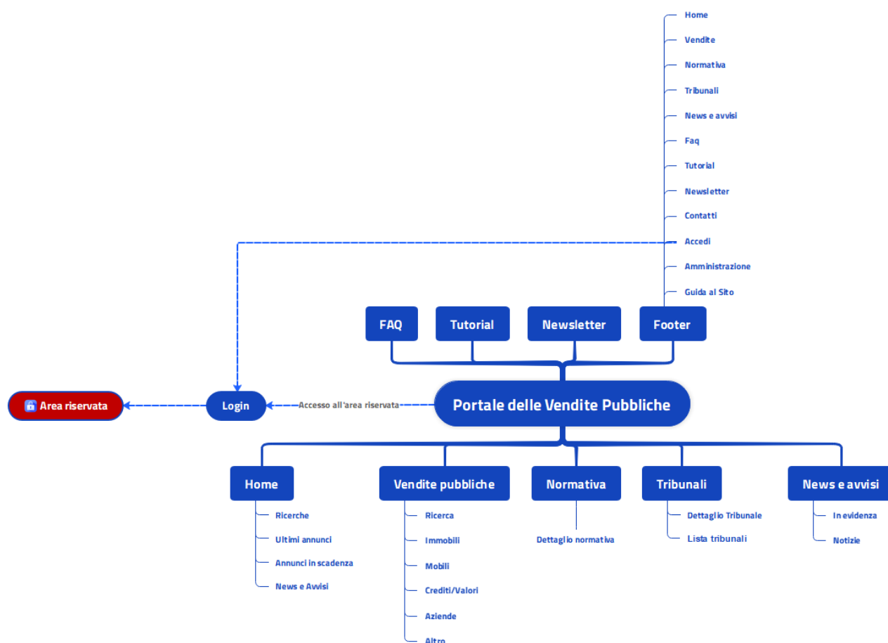
Figure 5 - Architettura dell'Informazione del Portale
