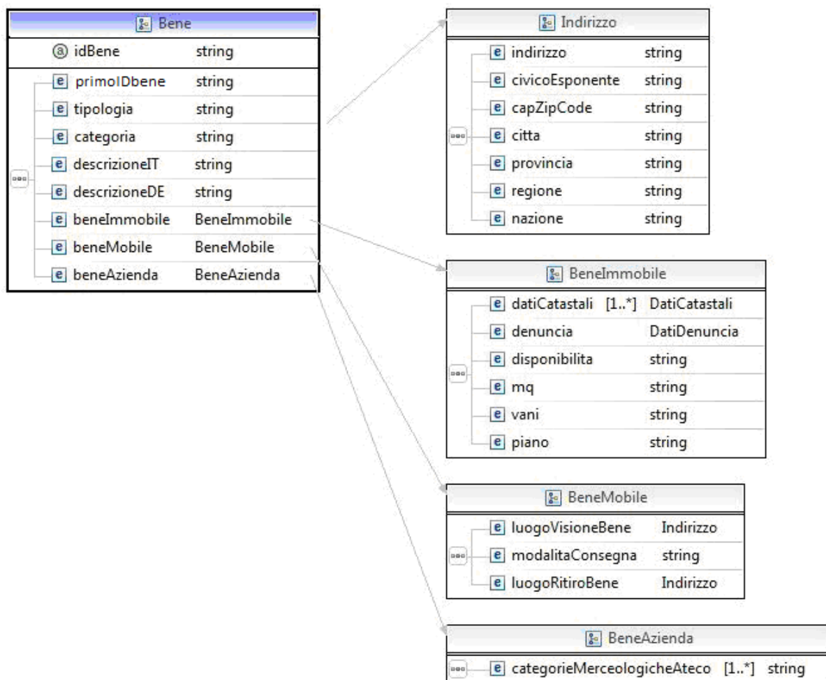
Figure 15 Struttura Bene
