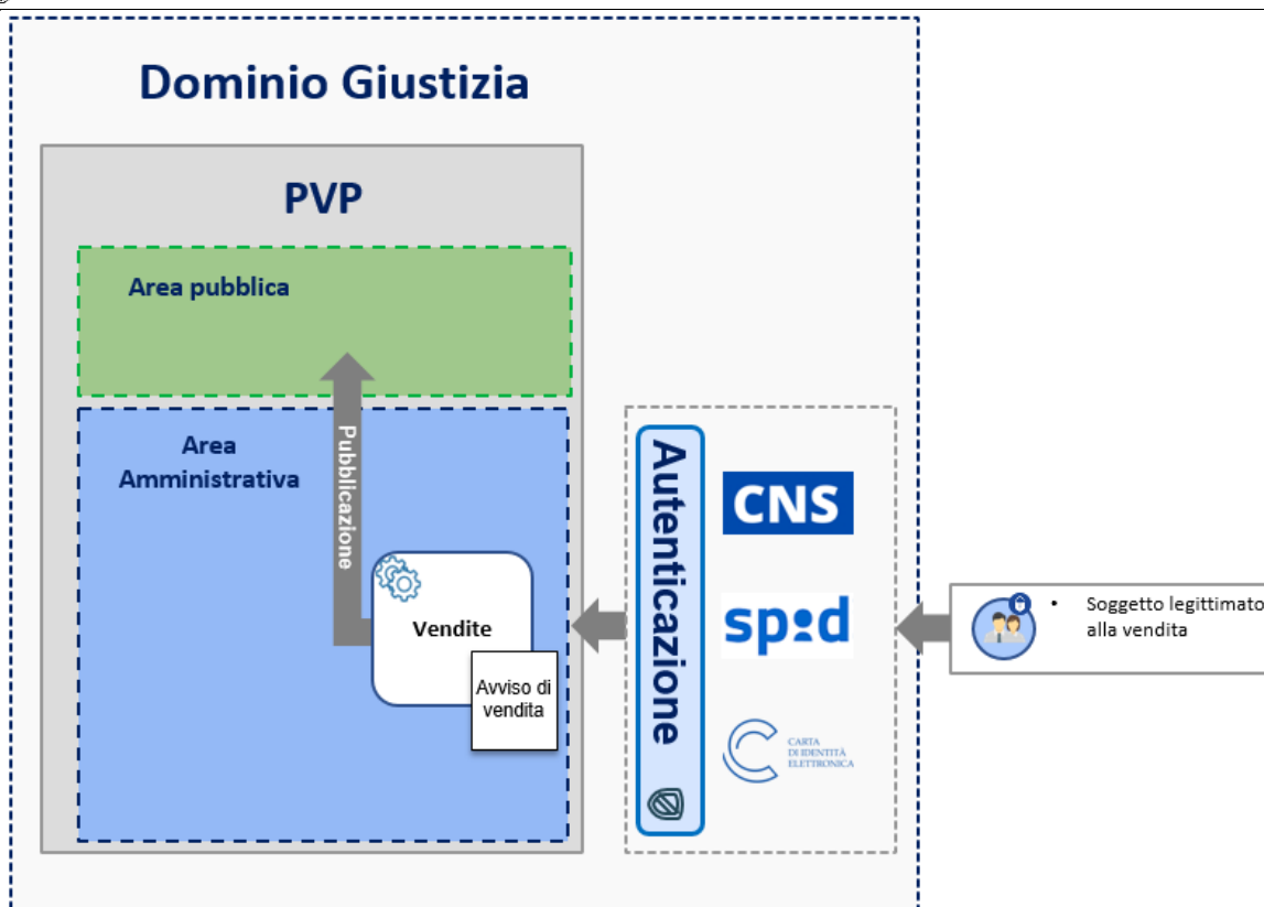
Figura 2 - Nuova inserzione
