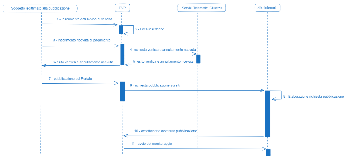
Figura 8 Flusso di trasmissione avviso di vendita
