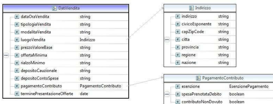
Figure 16 Struttura Dati Vendita
