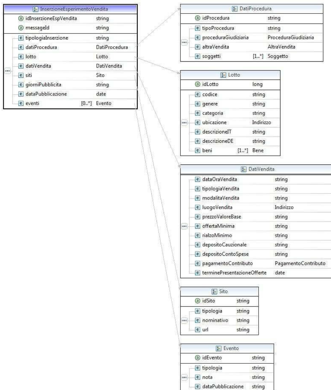
Figure 12 Relazione Inserzione Esperimento Vendita e le altre strutture
