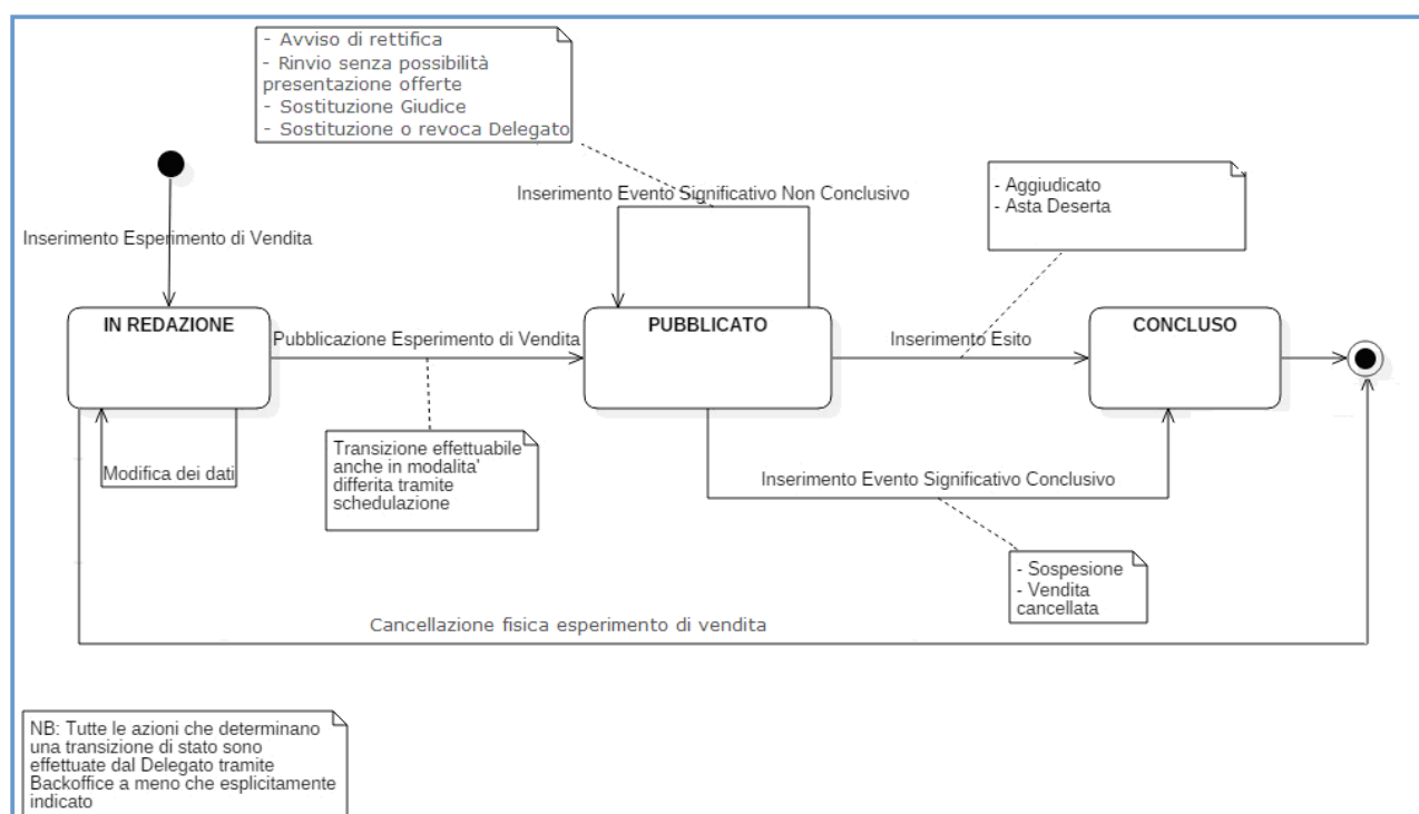
Figure 6 Diagramma degli stati dell'avviso di vendita
