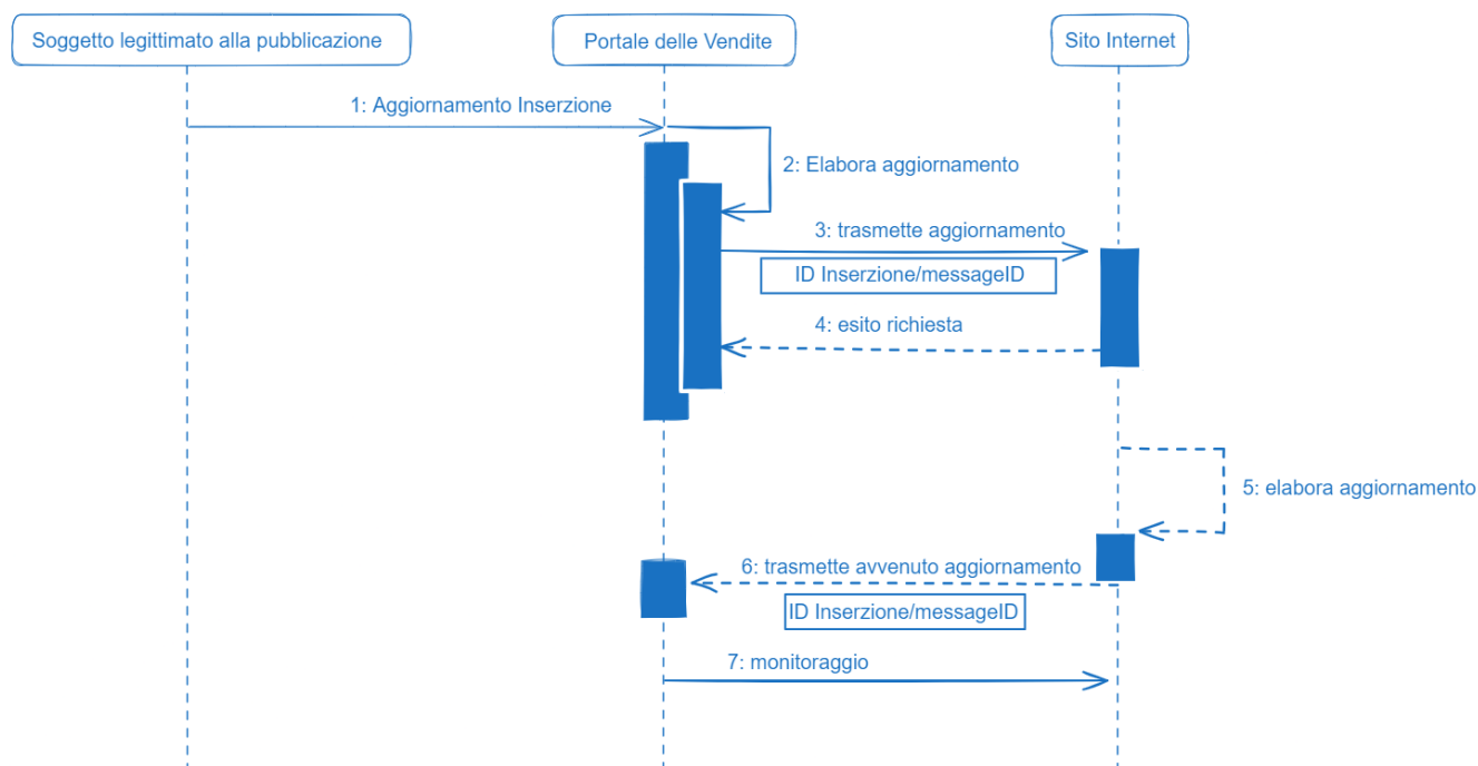
Figure 9 Flusso di trasmissione modifica avviso di vendita
