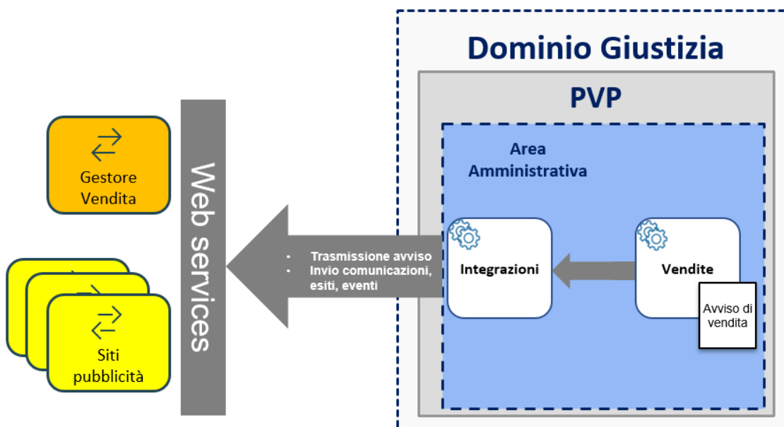
Figura 3 Trasmissione avvisi ai Siti Internet
