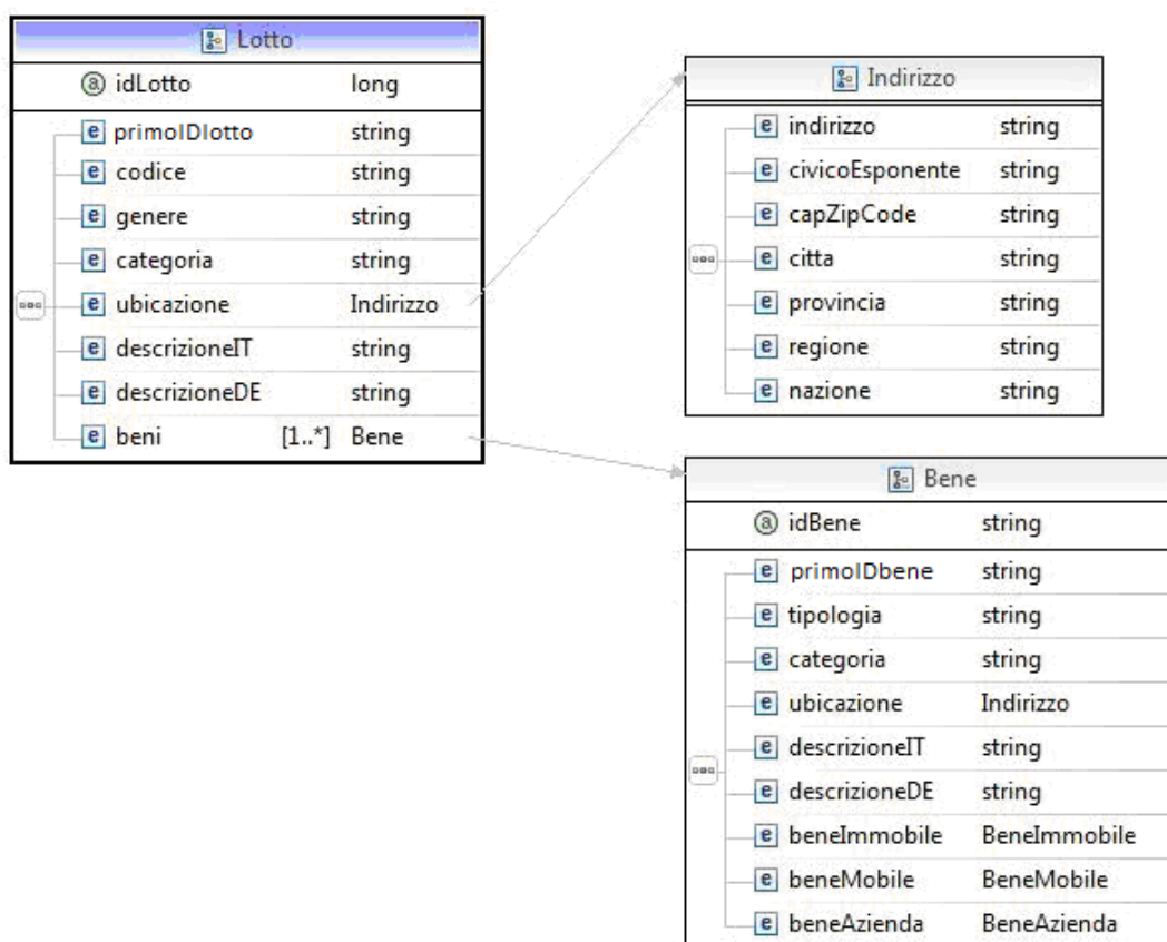
Figure 14 Struttura Lotto
