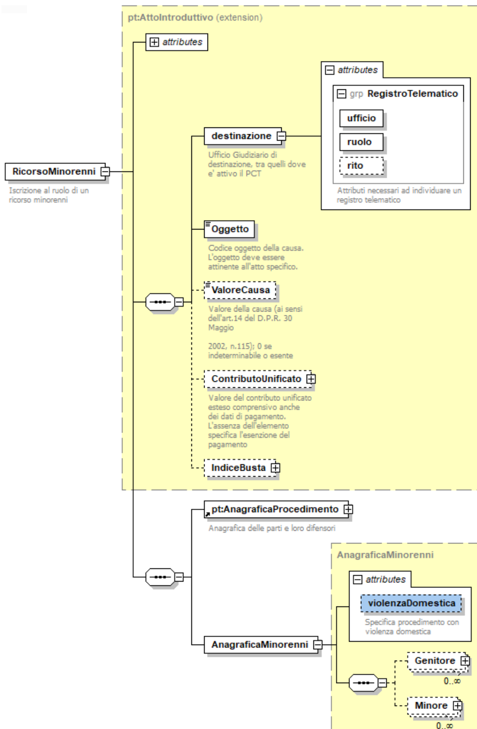
Figura 3 - Specifica di procedimento con "Violenza Domestica"
