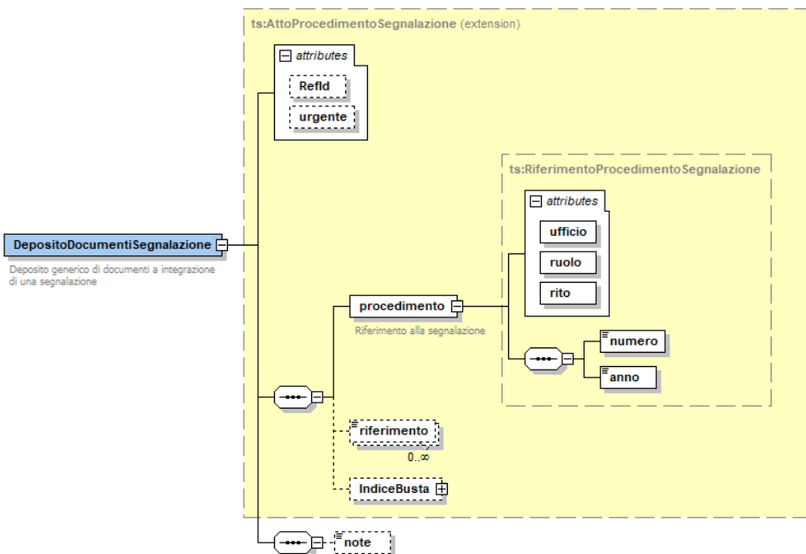
Figura 1 - Nuovo atto "DepositoDocumentiSegnalazione"
